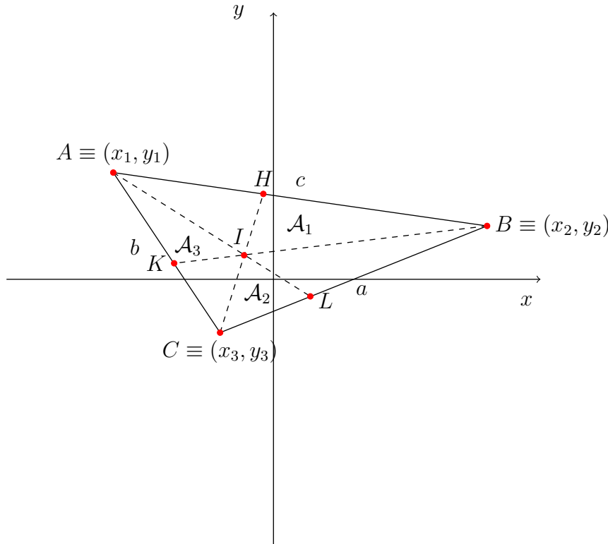
Figura 1: Incentro I del triangolo
